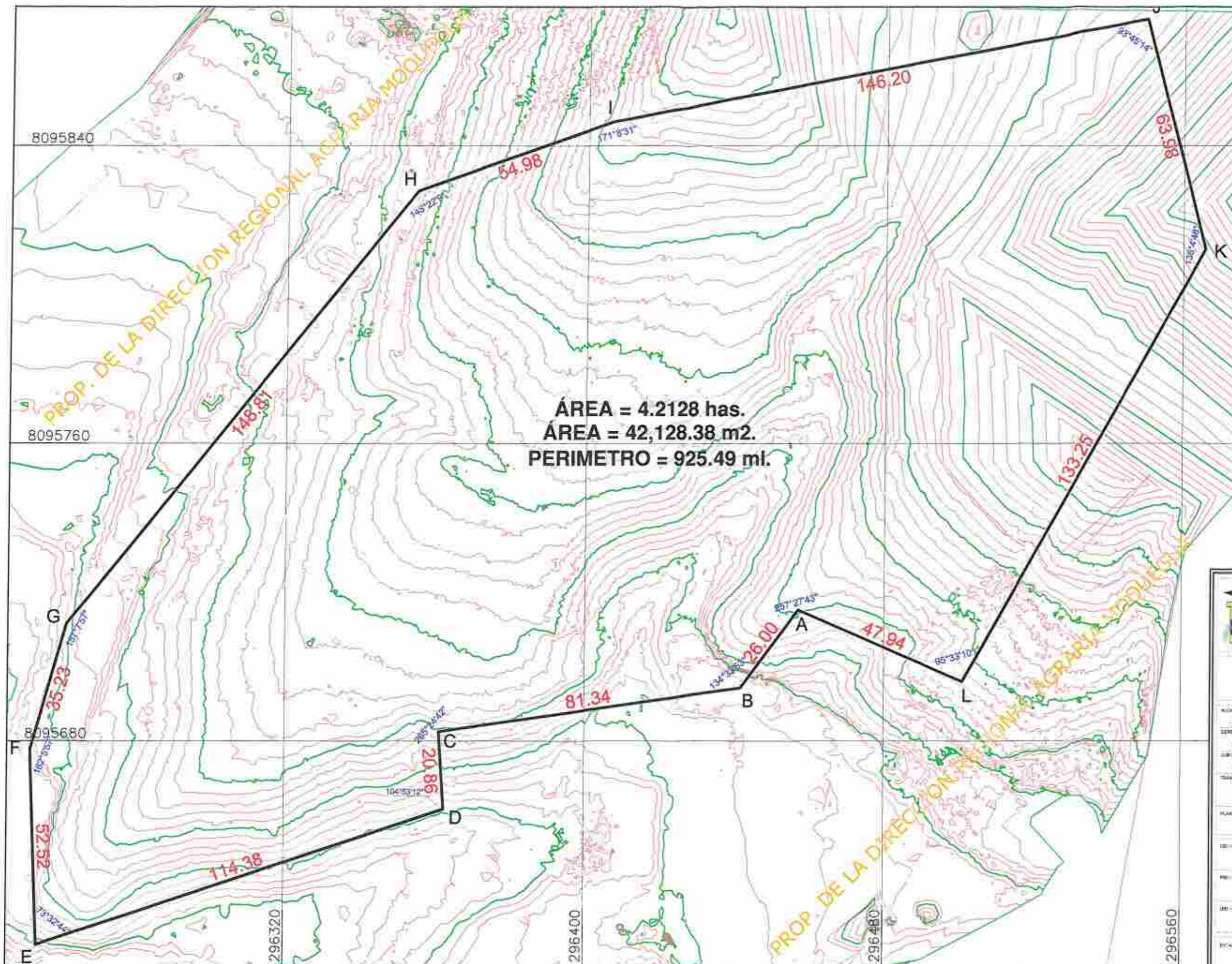
PLANO TOPOGRAFICO ESC:1:1,000
