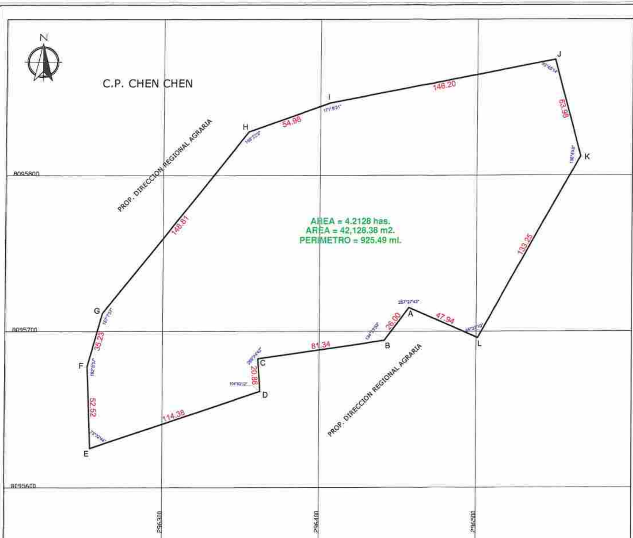
PLANO PERIMÉTRICO ESC: 1:1,000
