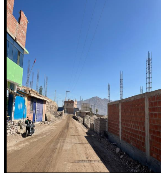
FIG. N°08: RELLENO, NIVELACIÓN Y COMPACTACIÓN CON MATERIAL PROPIO PREPARADO
